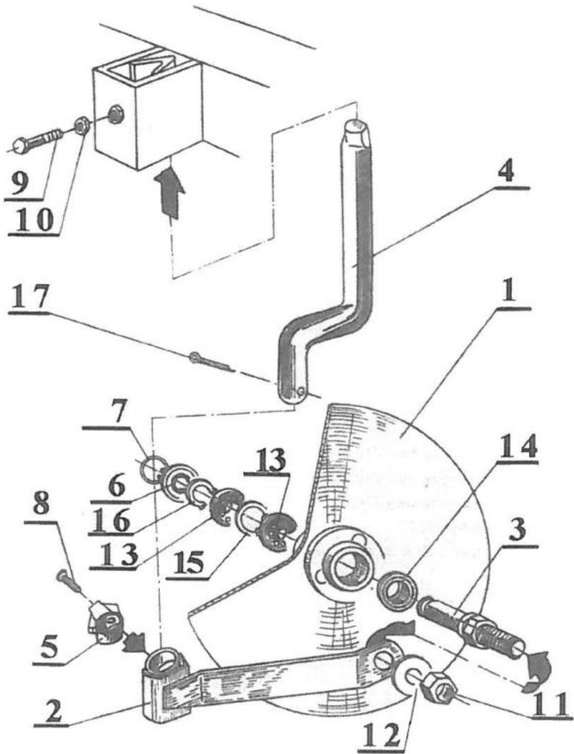
Дисковый (черенковый) нож (Таблица 4)
