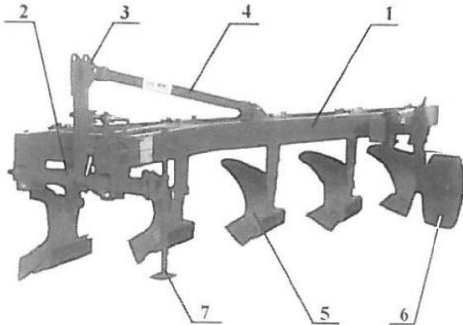
Рис. 2. Плуг подвесной 5-рядный Uo18
