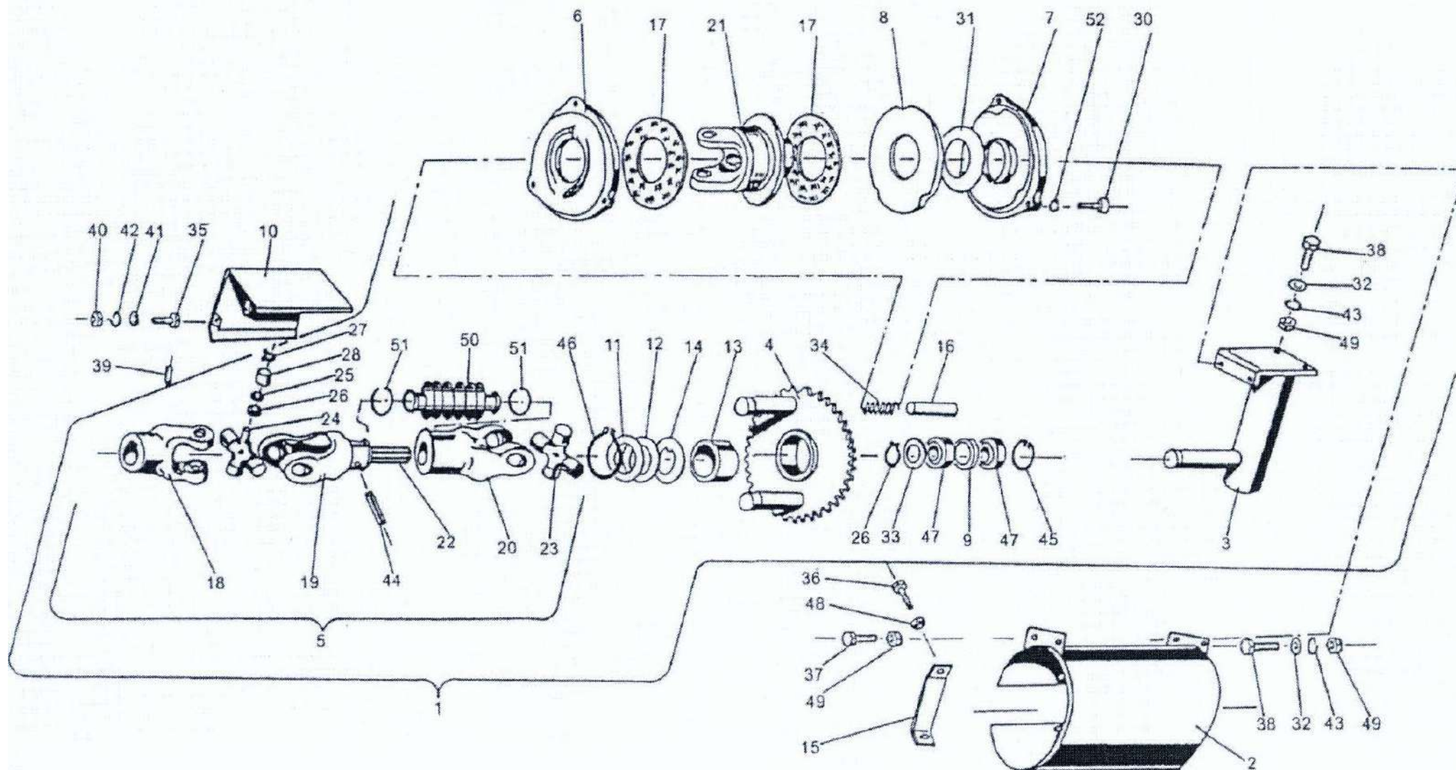
Tablica 19 Zespól 130 - Napęd podbieracza
